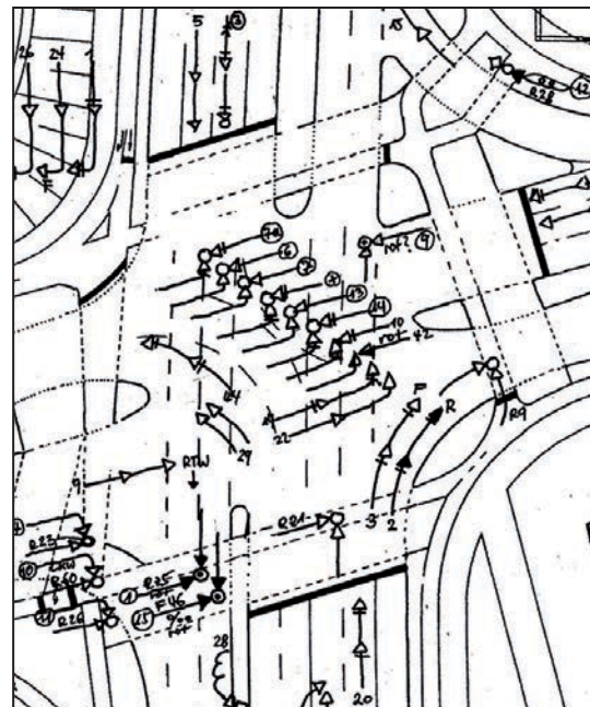
Abbildung 9: Beispiel einer Unfallhäufung durch fehlende Phase für Linksabbieger (Linksabbieger mit Gegenverkehr)
