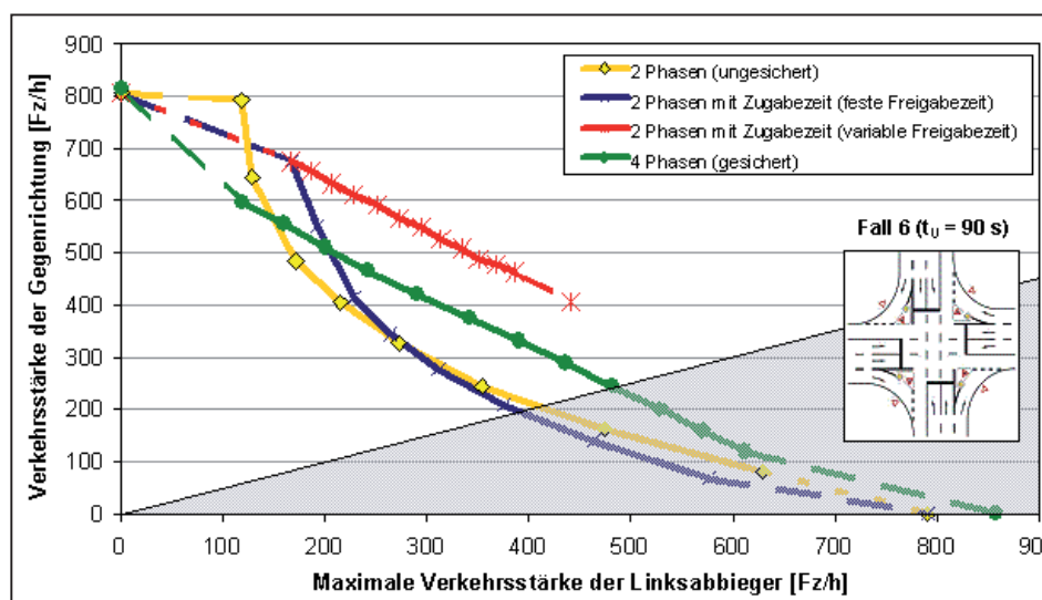
Abbildung 1: Vergleich des Einflusses eines konfligierenden Linksabbiegers bei unterschiedlichen Steuerungsverfahren für den Linksabbiegeverkehr auf die maximale Verkehrsstärke der übergeordneten Geradeausfahrer für große Kreuzungen mit Dreiecksinseln für eine Umlaufzeit von 90 s
