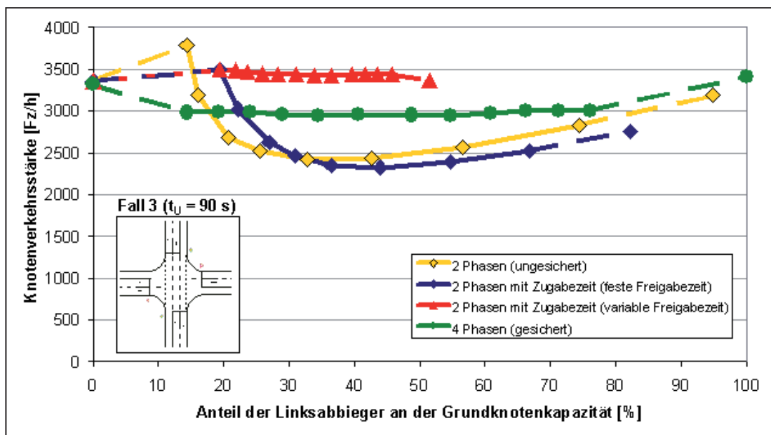
Abbildung 6: Knotenverkehrsstärke bei verschiedenen Steuerungsformen für mittlere Kreuzungen für eine Umlaufzeit von 90 s
