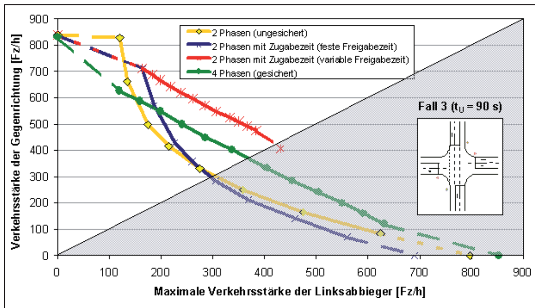
Abbildung 5: Vergleich des Einflusses eines konfigrierenden Linksabbiegers bei unterschiedlichen Steuerungsverfahren für den Linksabbiegeverkehr auf die maximale Verkehrsstärke der übergeordneten Gegenrichtung für mittlere Kreuzungen für eine Umlaufzeit von 90 s
