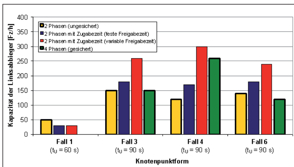
Abbildung 7: Kapazitäten der Linksabbieger bei einer Gegenverkehrsstärke von 600 Fz/(h*Fahrstreifen) für unterschiedliche Steuerungsvarianten der Linksabbieger und Knotenpunktformen – ein Ergebnis der Simulationsläufe
