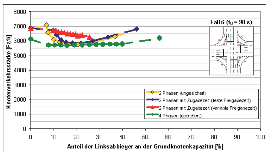
Abbildung 2: Knotenverkehrsstärke bei verschiedenen Steuerungsformen für große Kreuzungen mit Dreiecksinseln (Fall 6) für eine Umlaufzeit von 90 s
