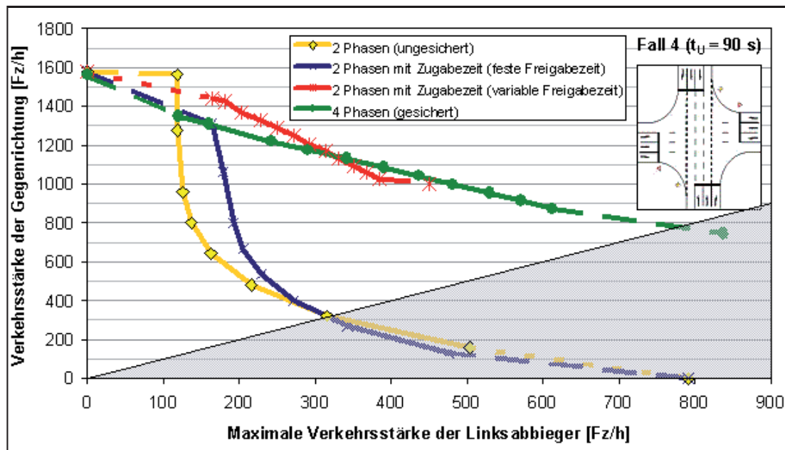
Abbildung 3: Vergleich des Einflusses eines konfigurierenden Linksabbiegers bei unterschiedlichen Steuerungsverfahren für die maximale Verkehrsstärke der übergeordneten Gegenrichtung für große Kreuzungen ohne Dreiecksinseln (Fall 4) für eine Umlaufzeit von 90 s
